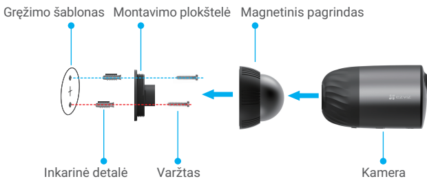
1 pav. Tvirtinimas naudojant magnetinį pagrindą
