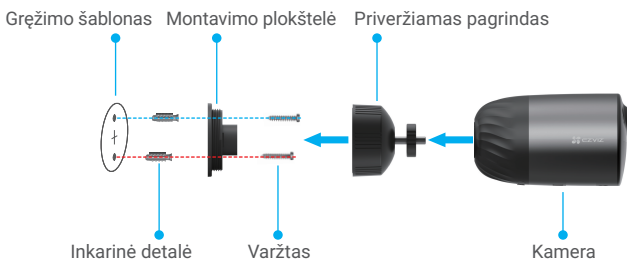
2 pav. Tvirtinimas naudojant priveržiamą pagrindą
